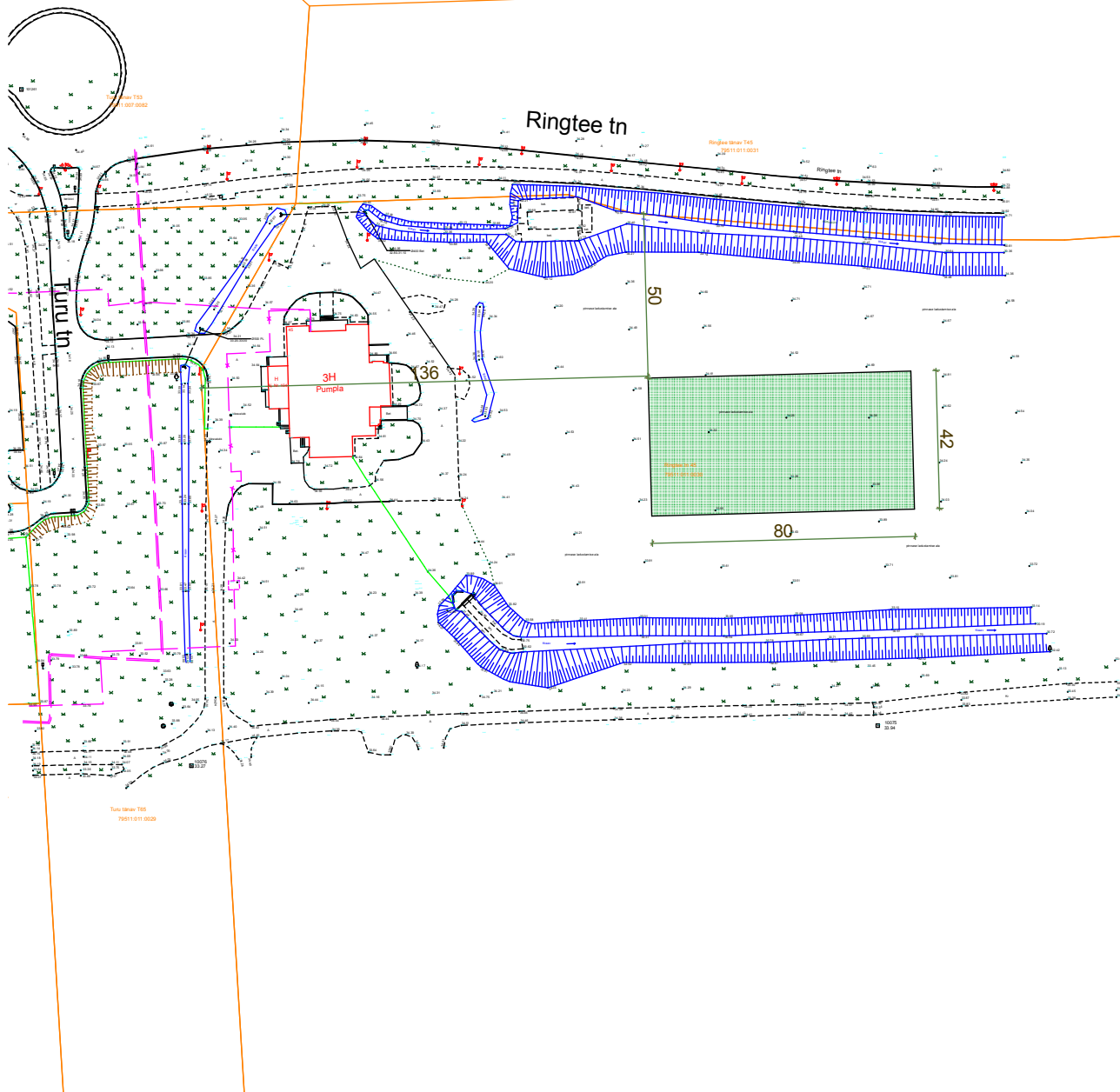
Lisa. Ehitusala skeem 1:2000. Ringtee tn 45 PTH-16-002
